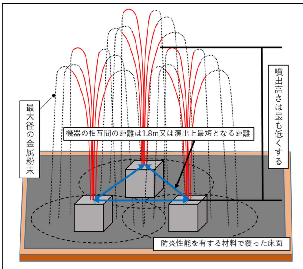
【図 2】 防災性能を有する材料及び床材への熱影響試験方法
