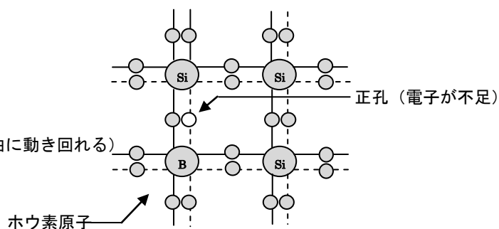
図2-4 p型半導体
