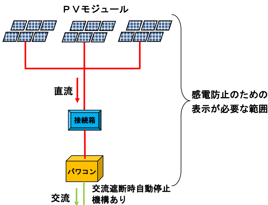
図7－13 感電防止のための表示が必要な範囲
