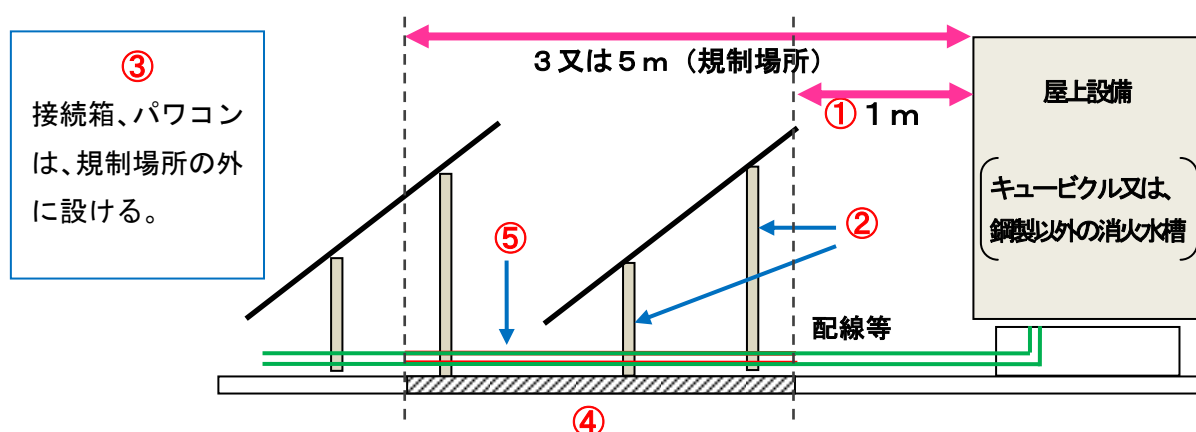
図 7 - 1 2 規制場所における P V モジュールの施工（断面図）
