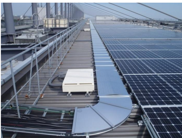
写真 7-17 表示が緩和される例 (PVモジュールと近接している配線、ケーブルラック、接続箱)
