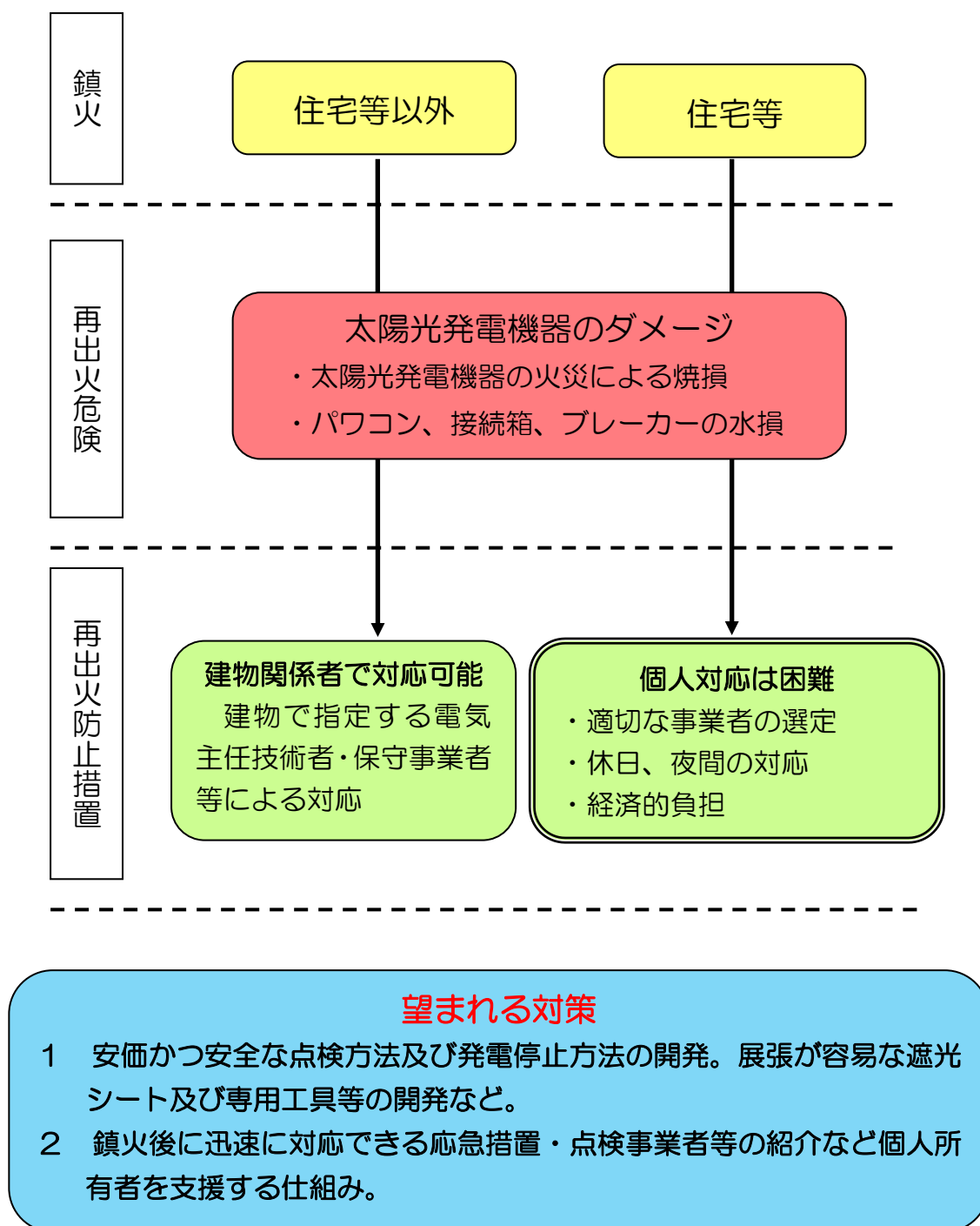
図 7 - 1 8 火災鎮火後の再出火防止対策
