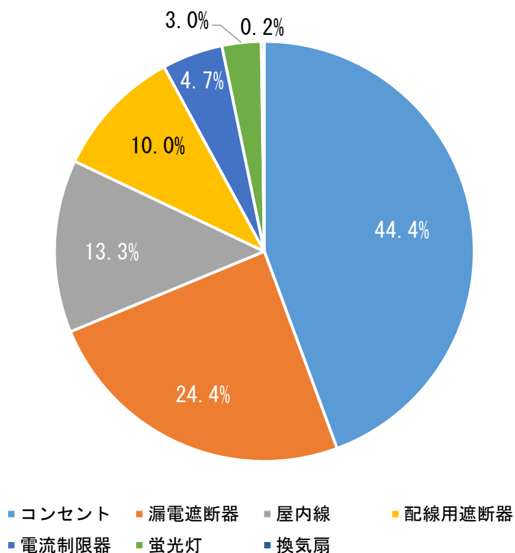
図 2－5 3 発火源別 件数・割合 建築設備 経過＝金属接触部過熱
