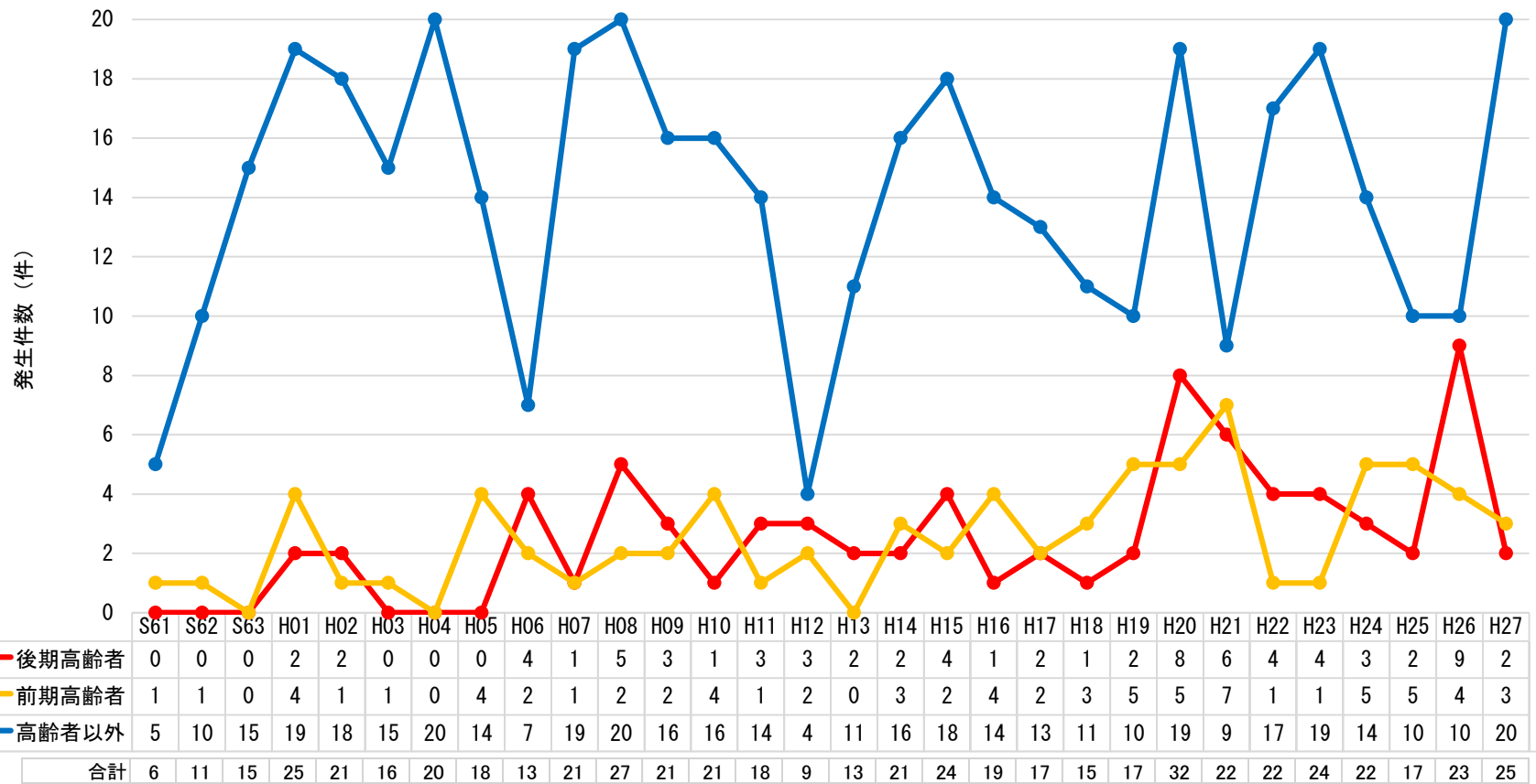
図 2 - 2 8 行為者年齢区分件数 発火源＝コード
