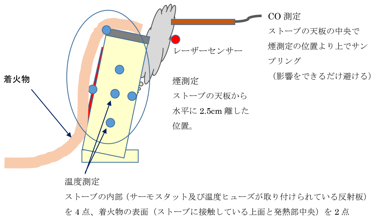
図 5 - 1 測定点のイメージ
