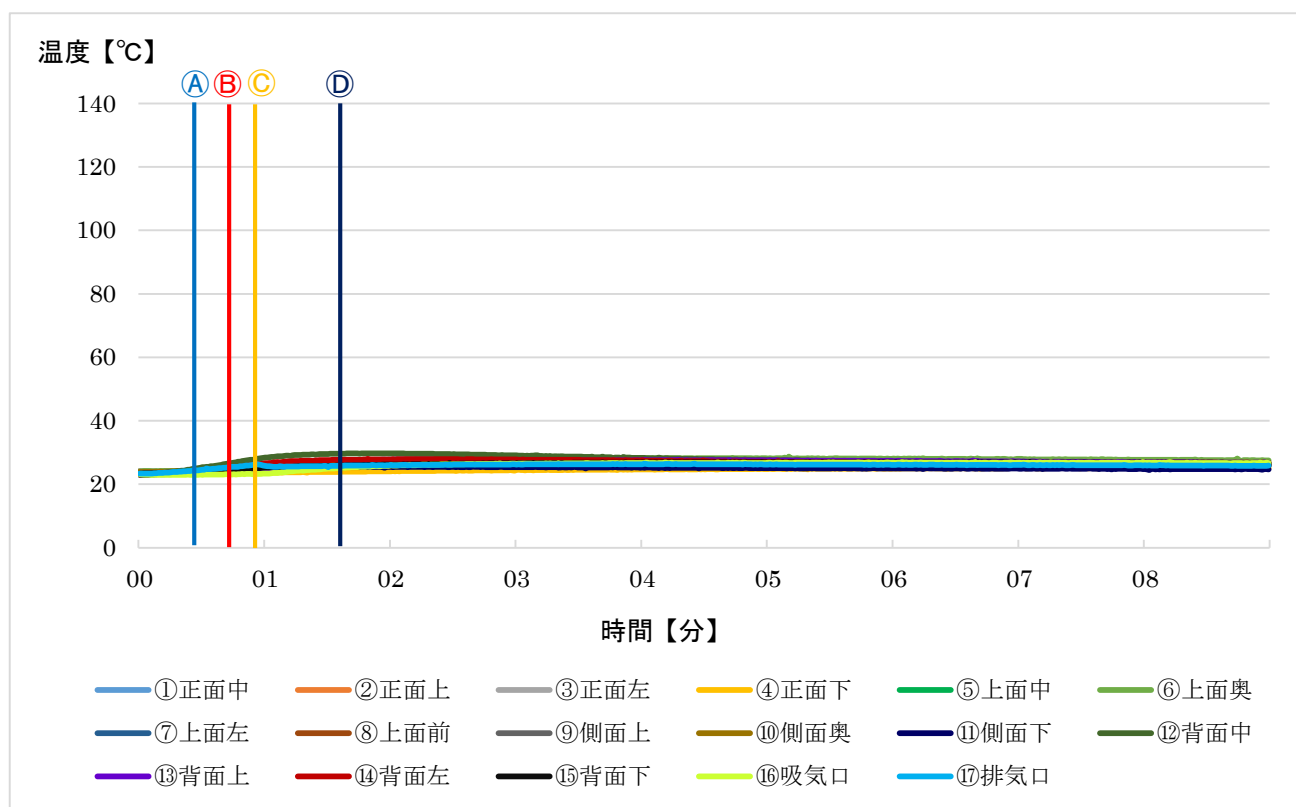
図4-41 メーカー推奨の電子レンジ停止による消火実験温度推移
