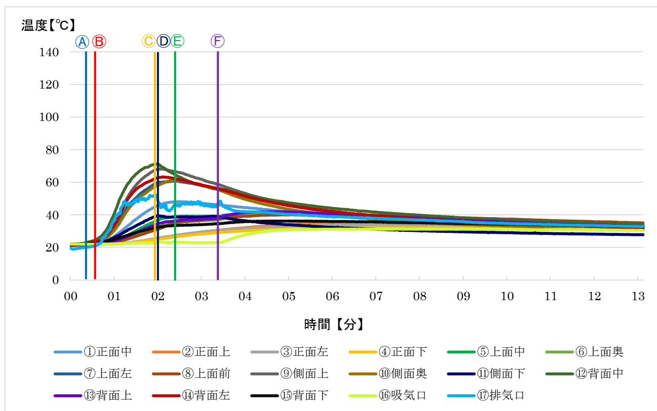
図4-25 消火器による吸気口への消火実験温度推移
