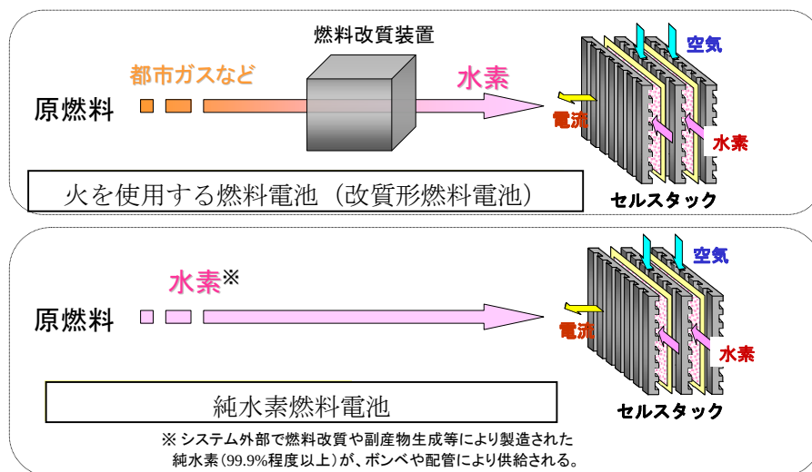
図 2.1.1-2 燃料改質装置の有無による分類
