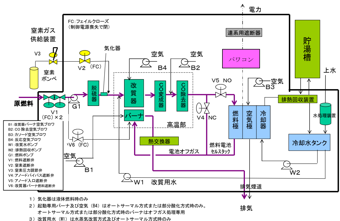
図 2.1.2-2 火を使用する燃料電池（固体高分子形）(PEFC) のシステムフロー図
