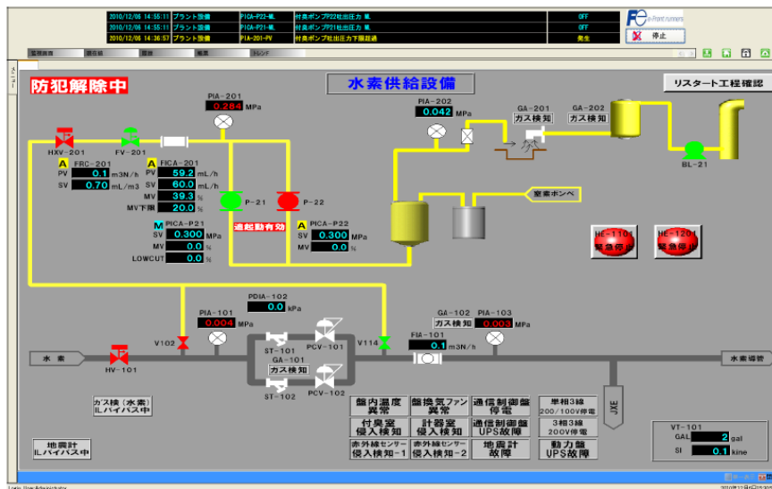
図 2. 2. 2. 3-11 水素供給設備の監視制御
