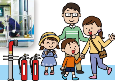
起震車体験
