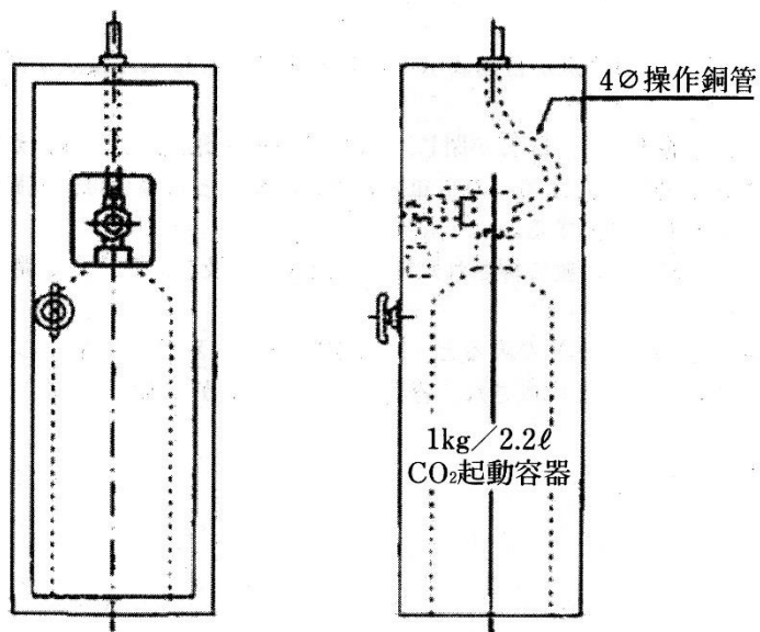
不活性ガス消火設備の起動容器例
