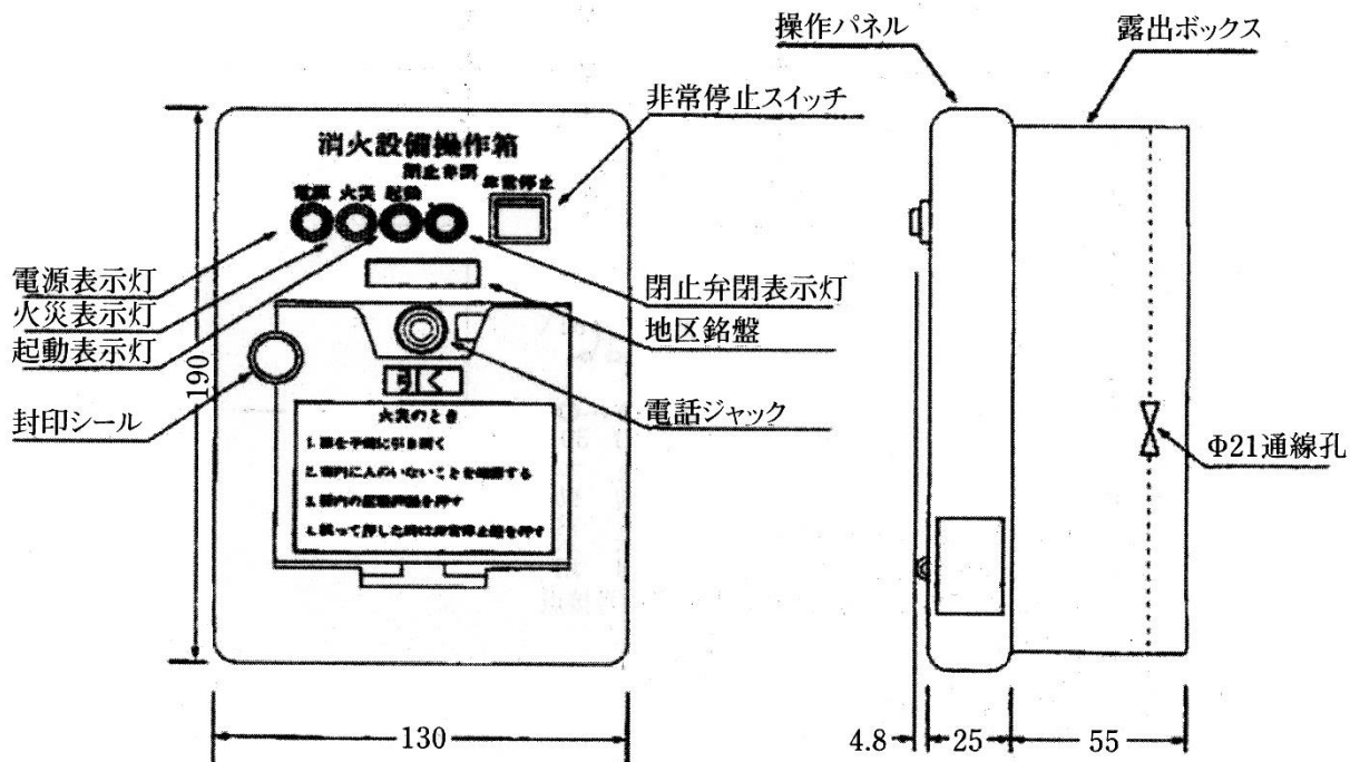
不活性ガス消火設備の操作箱の例
