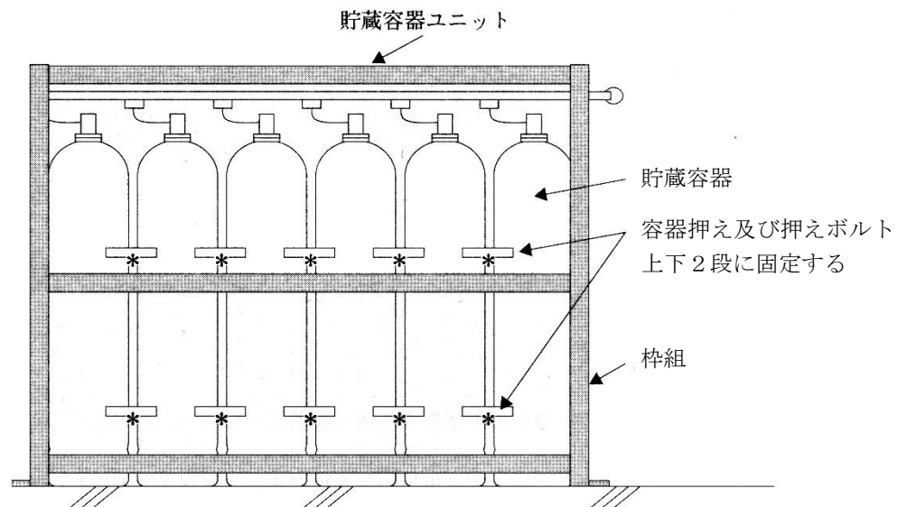
貯蔵容器の耐震措置例 第6－1図
