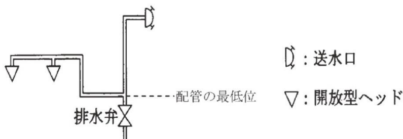
別図第20-1 排水弁の設置（例）
