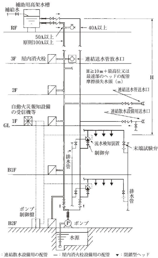
別図第 20-4 屋内消火栓設備兼用方式の配管と連結送水管の主管を兼用した場合の系統例
