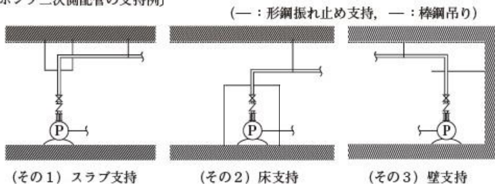
別図第21-3 非常用ELV設置対象の連結送水管の配管例
