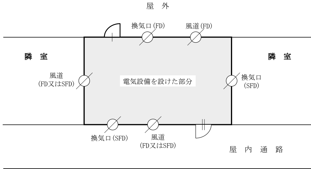
別図1 不燃区画された部分の例
