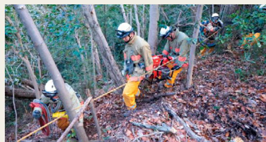
▲ 可搬式の小型消防ポンプ搬送
