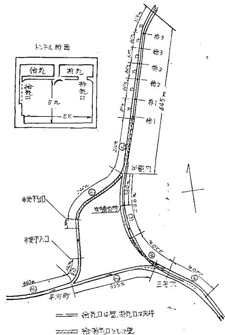
第1図 三宅坂インターチェンジの概況
