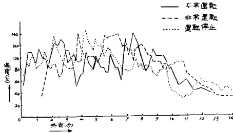
第5図 温度測定結果（火点天井下50cm）
