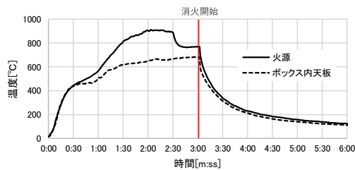
図 18 ボックス内消火時の温度変化
