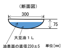
図4 油火災火源
