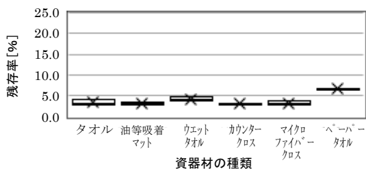
図11 トルエンの吸着のみによる各資器材の残存率
