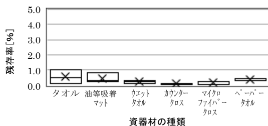
図9 水酸化ナトリウム水溶液（1 mol/L）の吸着のみによる各資器材の残存率
