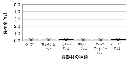
図5 塩酸（1 mol/L）のつまみ取りによる各資器材の残存率
