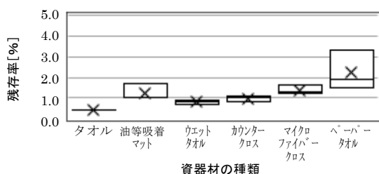
図2 塩酸（35%）の吸着のみによる各資器材の残存率
