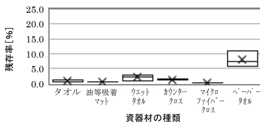
図 16 サラダ油のつまみ取りによる 各資器材の残存率
