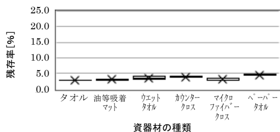
図 12 トルエンのつまみ取りによる 各資器材の残存率
