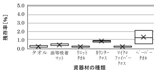
図3 塩酸（35%）のつまみ取りによる各資器材の残存率
