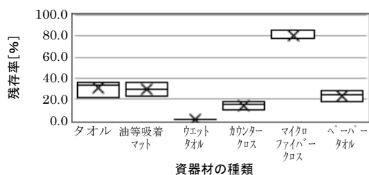
図7 水酸化ナトリウム水溶液（飽和）のつまみ取りによる各資器材の残存率
