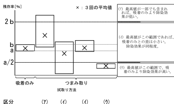
図 17 拭取り方法の違いによる評価の区分
