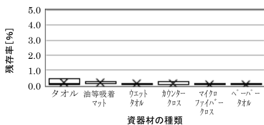
図10 水酸化ナトリウム水溶液（1 mol/L）のつまみ取りによる各資器材の残存率
