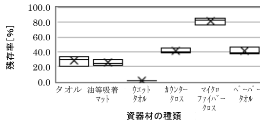
図6 水酸化ナトリウム水溶液（飽和）の吸着のみによる各資器材の残存率
