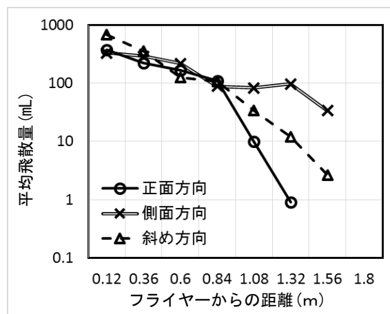
図 36 想定地震動によりフライヤーから各方向へ飛散した平均飛散量と距離の関係（溢流防止あり A）
