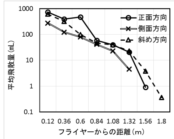
図 35 想定地震動によりフライヤーから各方向へ飛散した平均飛散量と距離の関係（溢流防止なし 3 回目）
