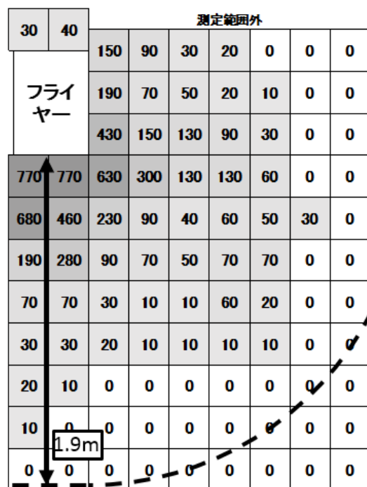
図 19 想定地震動によるフライヤーからの飛散量 (単位 mL、2 回目)
