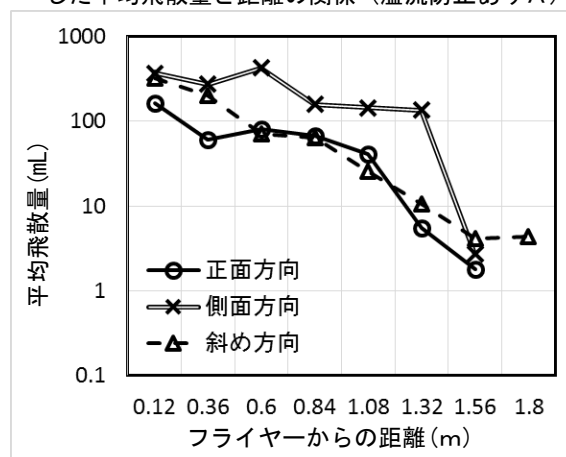
図 37 想定地震動によりフライヤーから各方向へ飛散した平均飛散量と距離の関係（溢流防止あり B）
