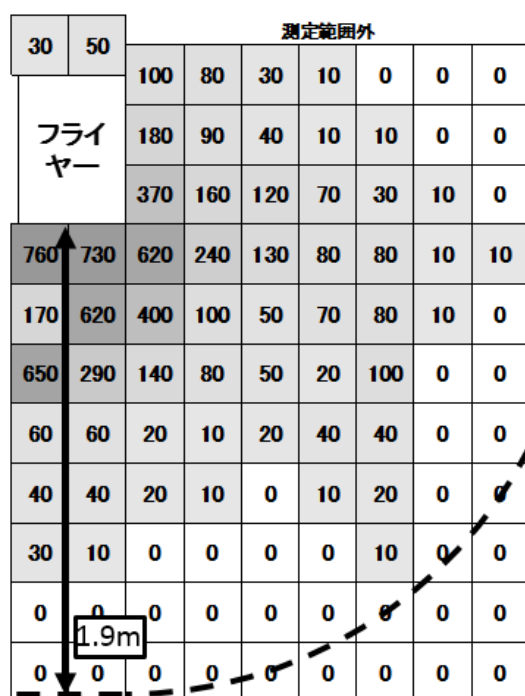
図 20 想定地震動によるフライヤーからの飛散量 (単位 mL、3 回目)
