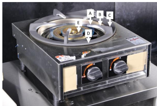
図 17 ガスこんろに対する油の滴下位置の設定
