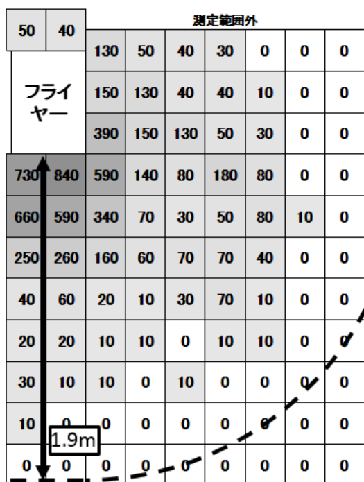
図 18 想定地震動によるフライヤーからの飛散量 (単位 mL、1 回目)
