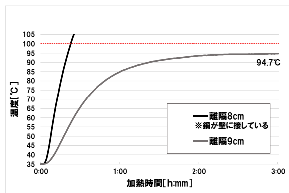
図 20 過大鍋ずらし加熱の温度上昇 （ケイカル板 10 mm 厚 2 枚張り）
