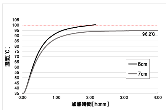
図 11 ケイカル板 10 mm厚+5 mm厚の温度上昇
