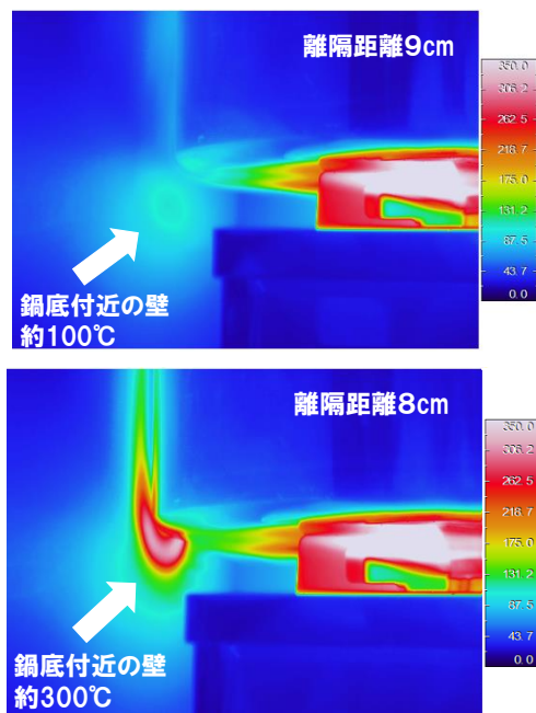
図 25 過大鍋ずらし加熱中の熱画像
