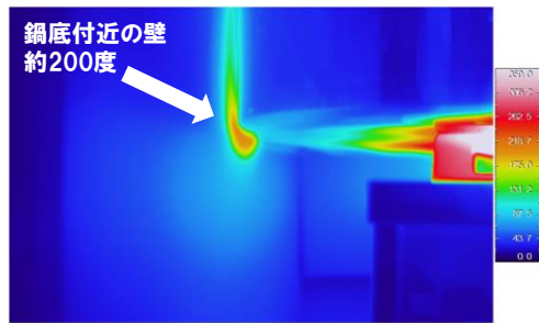
図 28 過大鍋ずらし検証②加熱中の熱画像
