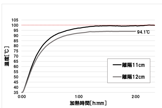
図 23 過大鍋ずらし加熱の温度上昇 (ケイカル板 5 mm厚 1 枚張り)
