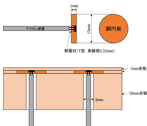
図4 温度測定点の構造
