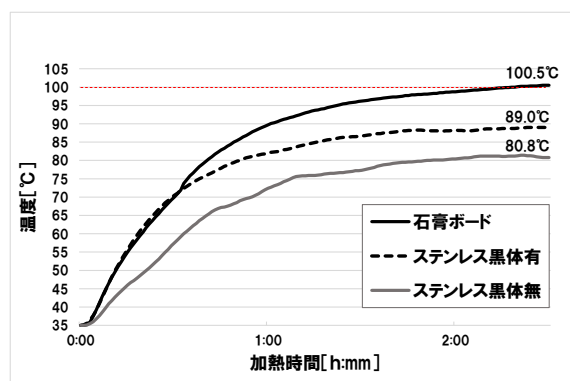
図 16 ステンレス仕上げの温度上昇比較
