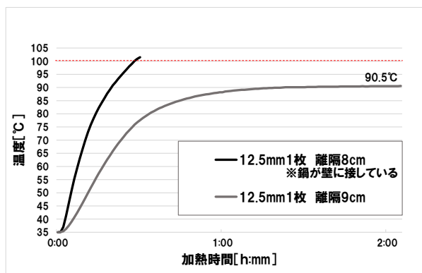
図 18 過大鍋ずらし加熱の温度上昇 （石膏ボード）
