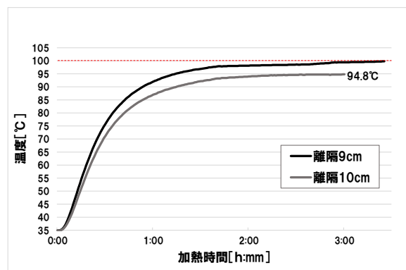
図 21 過大鍋ずらし加熱の温度上昇 （ケイカル板 10 mm 厚 + 5 mm 厚）
