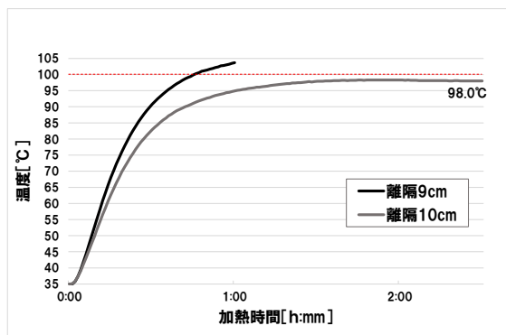
図 22 過大鍋ずらし加熱の温度上昇 (ケイカル板 10 mm厚 1 枚張り)
