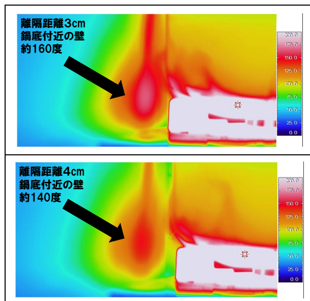
図8 石膏ボード仕上げ加熱中の熱画像
