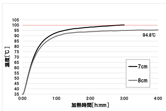
図 12 ケイカル板 10 mm厚 1 枚張りの温度上昇
