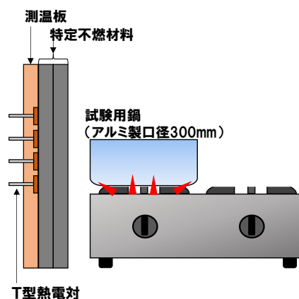
図5 通常鍋加熱検証イメージ
