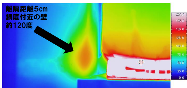
図 14 ケイカル板仕上げ加熱中の熱画像 (離隔距離 5 cm)
