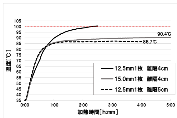
図9 石膏ボード 12.5 mm厚 1枚張り及び 15.0 mm厚 1枚張りの温度上昇
