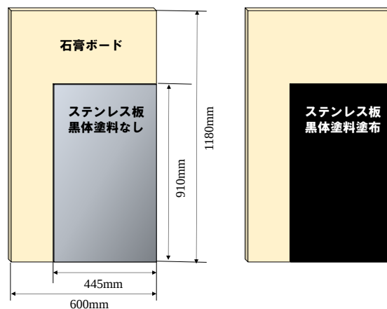
図 15 ステンレス板仕上げイメージ
