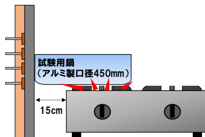
図 26 過大鍋ずらし検証②イメージ
