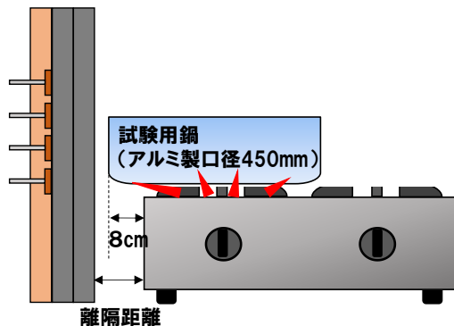
図 17 過大鍋ずらし検証①イメージ
