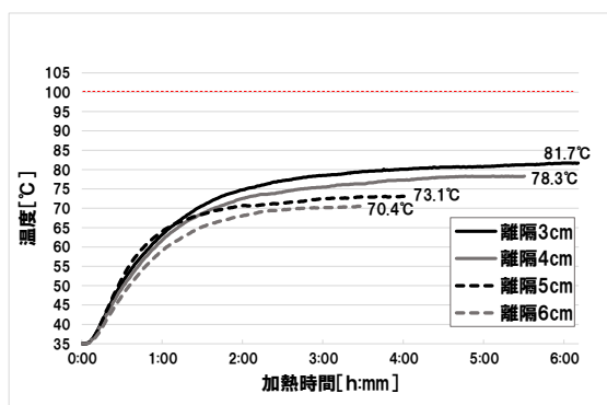
図6 石膏ボード 12.5 mm厚 2枚張りの温度上昇
