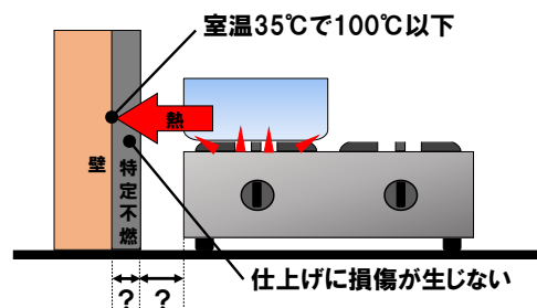
図 1 検証イメージ
