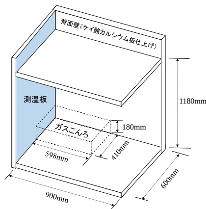
図3 測温台の外形寸法
