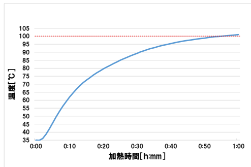
図 27 過大鍋ずらし検証②の温度上昇
