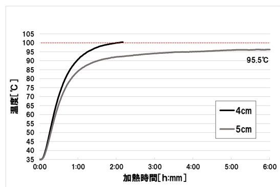
図10 ケイカル板 10mm厚 2枚張りの温度上昇
