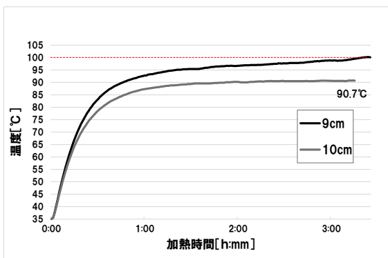
図 13 ケイカル板 5 mm厚 1 枚張りの温度上昇
