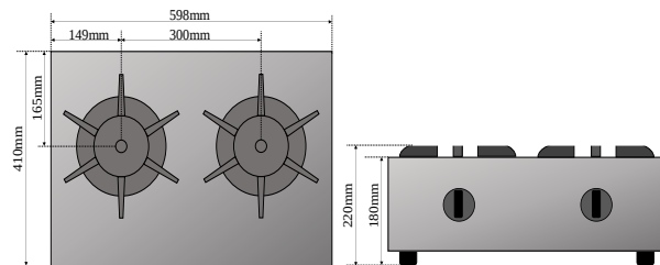
図 2 ガスこんろ外形寸法（左：平面図、右：立面図）
