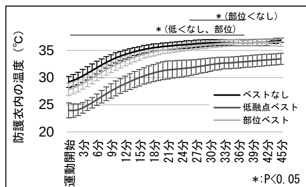
図 14 冷却部位別の毒劇物防護衣内温度
