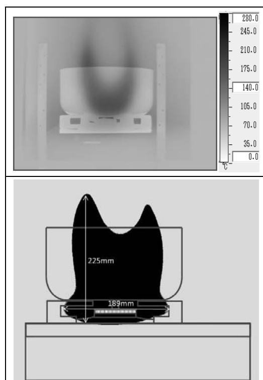
図9 ステンレス板防熱板裏面の熱環境
