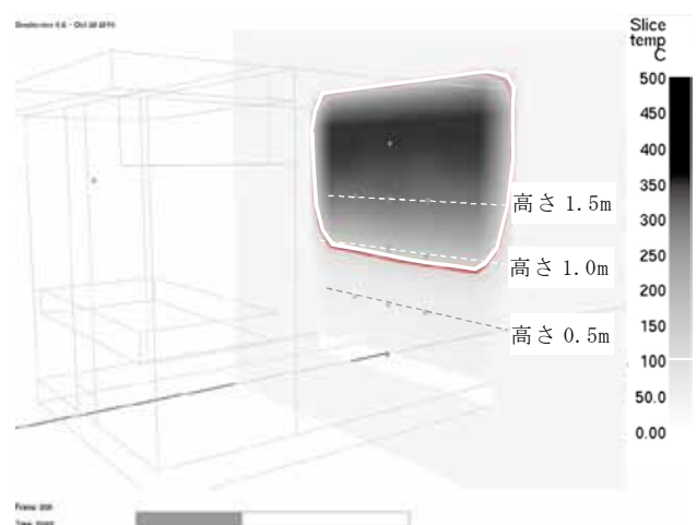
図19 短辺断面の熱環境の可視化及び等温線(100℃)の状況(時刻約13分30秒 施設温度計(中段)250℃)
