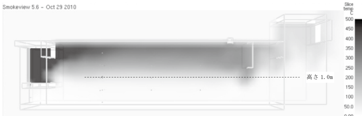
図 14 長辺断面の熱環境の可視化の状況（木質パレット 5 枚）（時刻約 4 分 30 秒）
