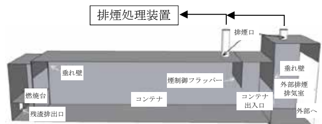
図1 当施設の構造
