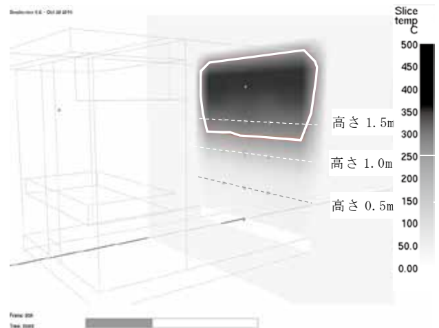
図17 短辺断面の熱環境の可視化及び等温線(250℃)の状況(時刻約13分30秒 施設温度計(中段)温度250℃)
