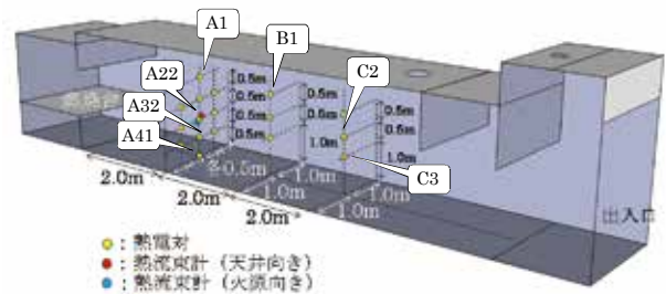
図 5 熱電対及び熱流束計の測定位置
