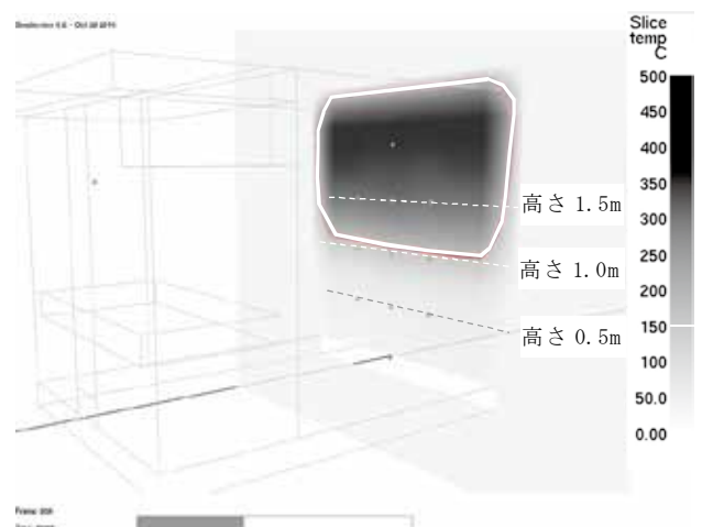
図18 短辺断面の熱環境の可視化及び等温線(150℃)の状況(時刻約13分30秒 施設温度計(中段)温度250℃)
