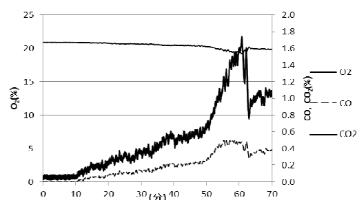
図 18 実験 3 発生ガスの濃度変化（口元付近）
