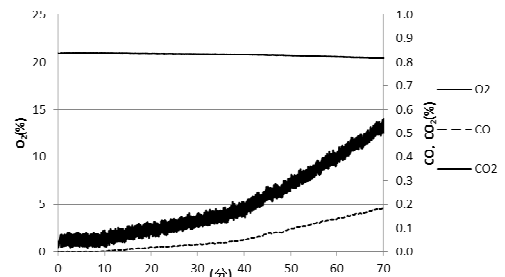
図 23 実験 6 発生ガスの濃度変化（天井付近）
