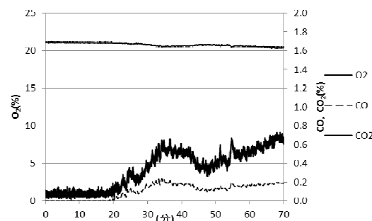
図 20 発生ガスの濃度変化（口元付近）
