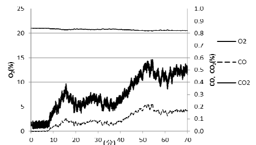
図 24 実験 6 発生ガスの濃度変化（口元付近）
