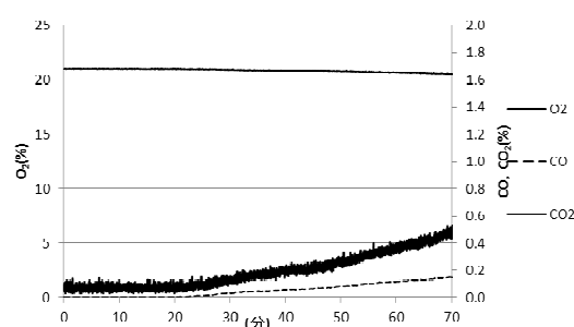
図 19 実験 4 発生ガスの濃度変化（天井付近）
