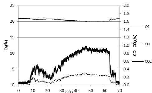
図 14 実験 1 発生ガスの濃度変化 (口元付近)
