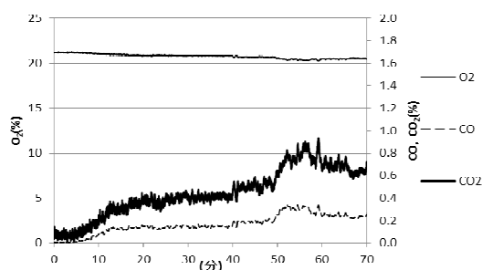
図 16 実験 2 発生ガスの濃度変化（口元付近）
