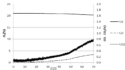
図 15 実験 2 発生ガスの濃度変化 (天井付近)
