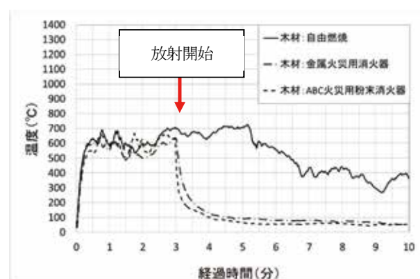
図2 木材の表面温度( T_1 )
