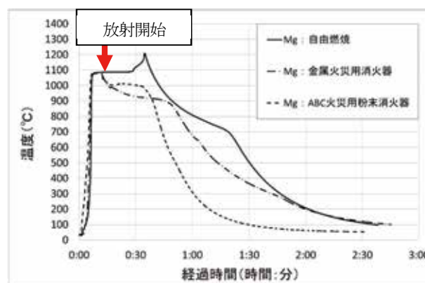
図1 マグネシウムの内部温度( T_m )
