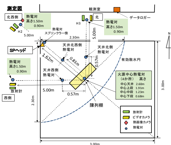
図4 平面図
