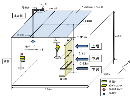
図3 立面図
