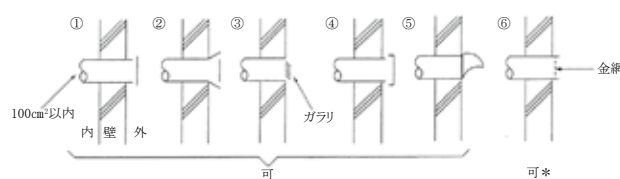
図6 防火設備とみなされる防火覆いの例 2)
