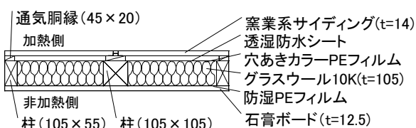
図 23 実験 No. 18 で使用した試験体断面図[mm]
