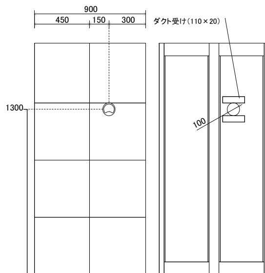
図 26 実験 No. 21～26 で使用した試験体正面図と内部[mm]
