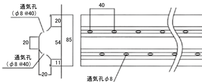
図 18 熱気止め材 [mm]
