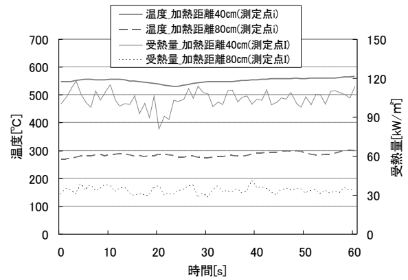
図 28 温度測定点 i、受熱量測定点 I 時系列データ
