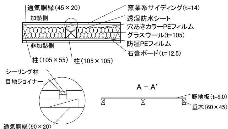
図9 試験体の全体像[mm]
