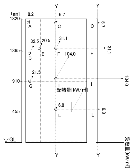
図 32 加熱距離 40 cm 受熱量分布
