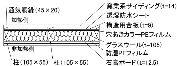
図 17 実験 No. 13 で使用した試験体断面図 [mm]
