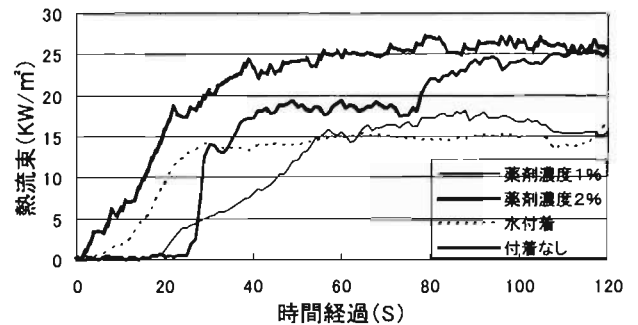
図10 合板表面上部の受熱量の変化
