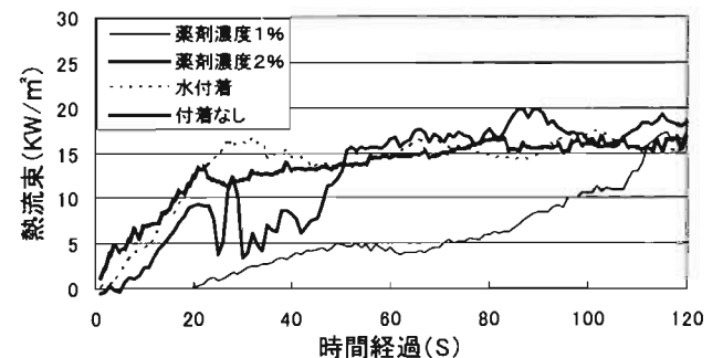
図11 合板表面下部の受熱量の変化
