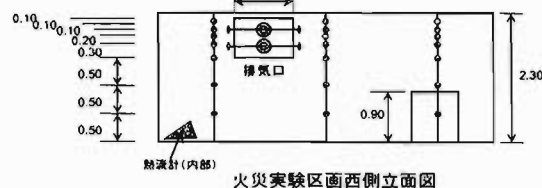
b) 立面図
