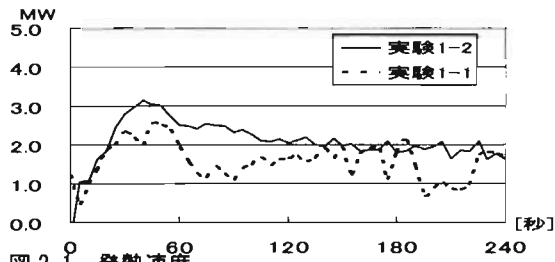
図 2-1 発熱速度
