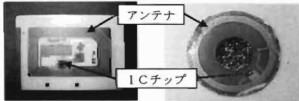
写真12 シート型ICタグのインレット
