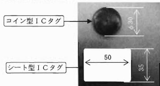
写真14 ICタグ
