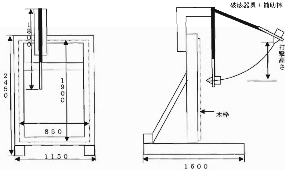
図1 実験装置
