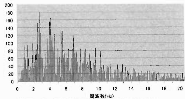
図9-2 資機材搬送の加速度周波数成分
