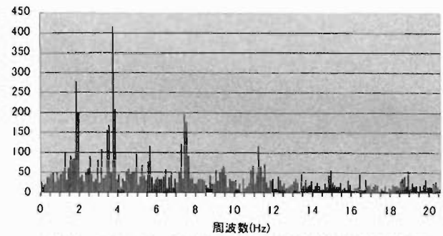
図8-2 ホースカーえい行の加速度周波数成分
