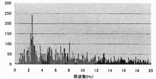
図10-2 救助活動の加速度周波数成分
