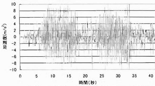
図8-1 ホースカーえい行の加速度波形
