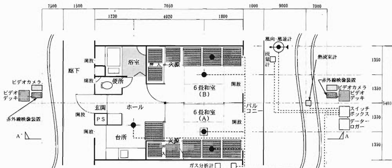
図4 測定機器等の配置図(平面図)
