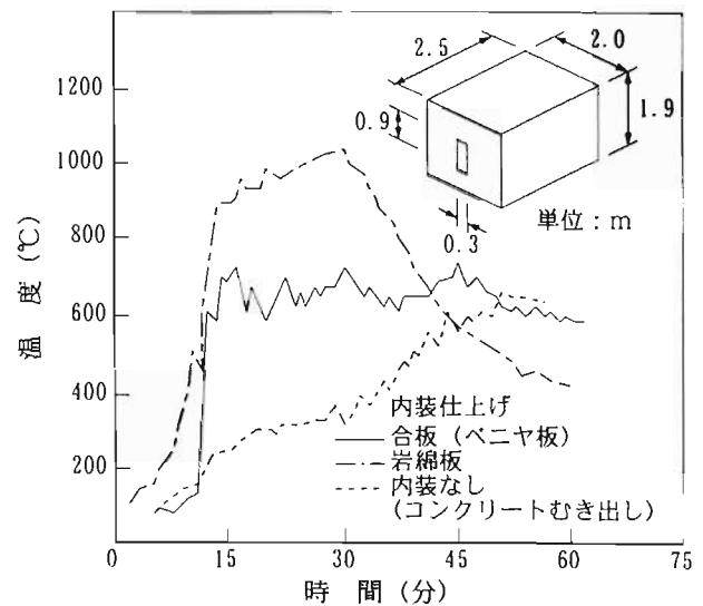
図15 内装の仕上げと火災温度
