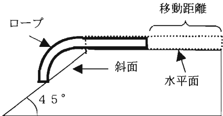
図 11 硬さ試験装置 (側面図)
