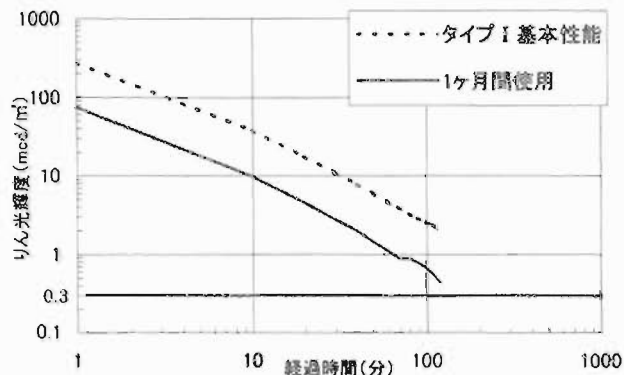
図 13 使用後の残光輝度
