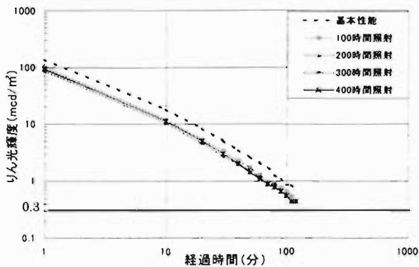
図 10 耐候性 (タイプⅡ)
