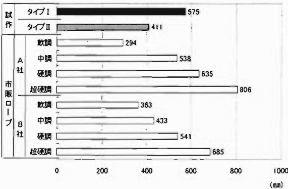
図 12 硬さ試験結果
