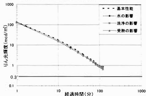
図 8 水・洗浄・受熱の影響 (タイプ II)
