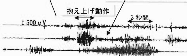
図 17 床上座位傷病者抱え上げ前後の筋電図波形(波形の位置は図 16 と同じ)
