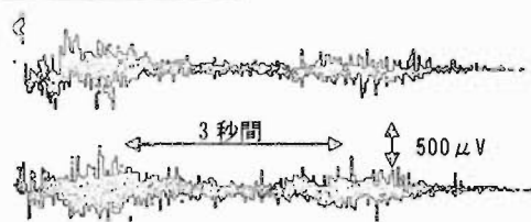
図 20 拾う動作時の腰部筋電図 (波形の位置は図 15 と同じ)
