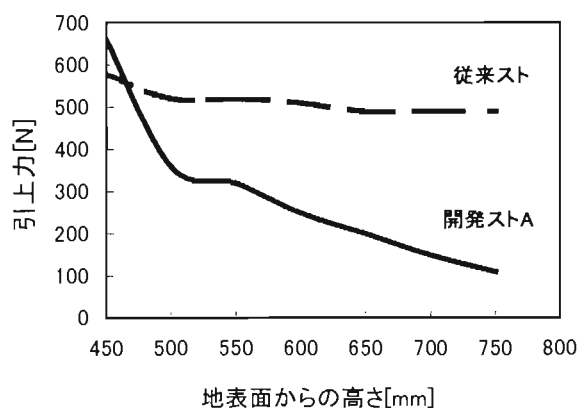
図3 引上力の比較(35kg荷重)
