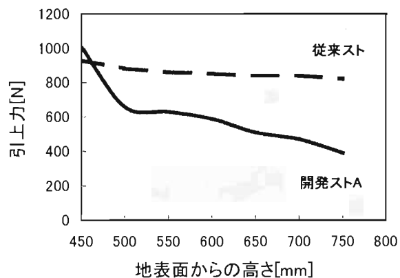
図4 引上力の比較(70kg荷重)
