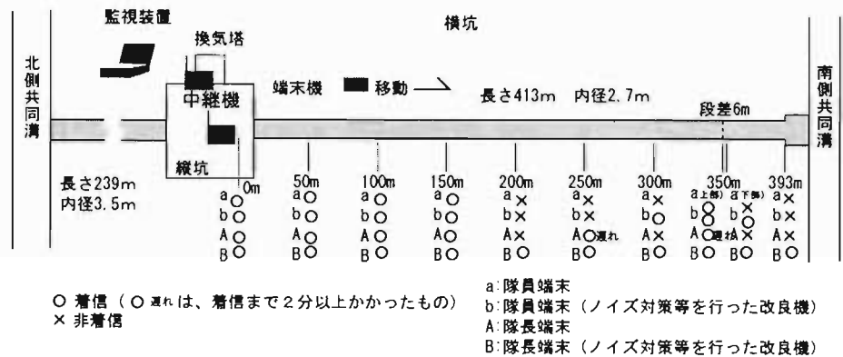
図 8 地下洞道実験結果 (平面図)
