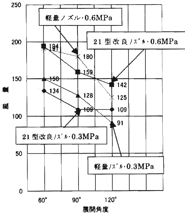
図3 展開角度と風量
