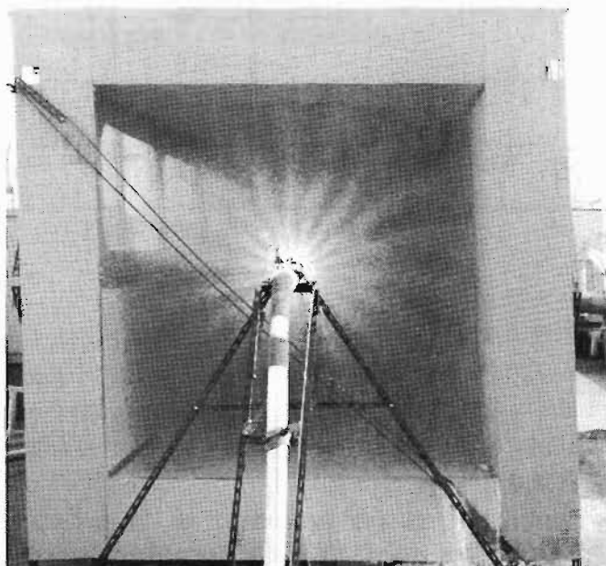
写真3 実験1の噴霧放水状況
