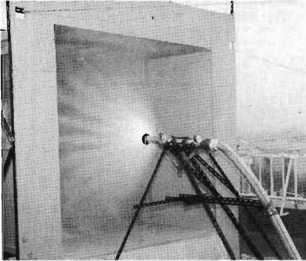
写真4 実験1の噴霧放水状況
