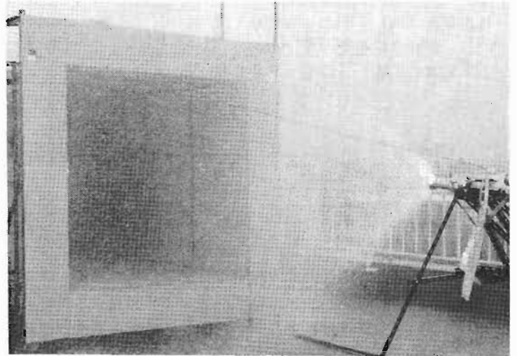
写真5 実験2の噴霧放水状況
