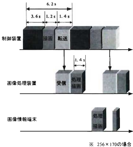
※ 256×170の場合 図13 視覚装置のタイムテーブル
