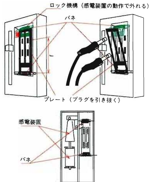
図5 機械バネ式 (直接起動方式)
