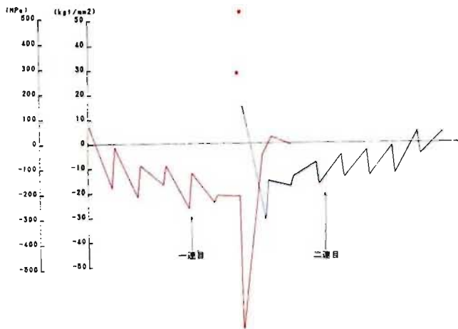
図8 65°架てい状態の応力測定結果 (7段目、3,234N (330kgf) 荷重時)
