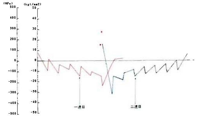
図 4 水平荷重状態の応力測定結果 (882 N (90kgf) 荷重時)
