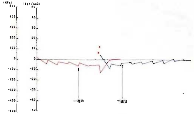
図6 65°架てい状態の応力測定結果 (7段目、882 N (90kgf) 荷重時)
