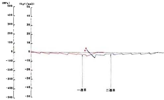
図5 水平荷重状態の応力測定結果 (自重のみの状態)
