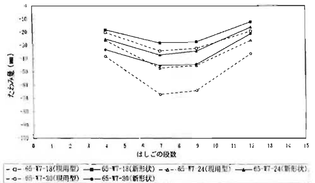
図7 65°架てい時のたわみ量の測定結果
