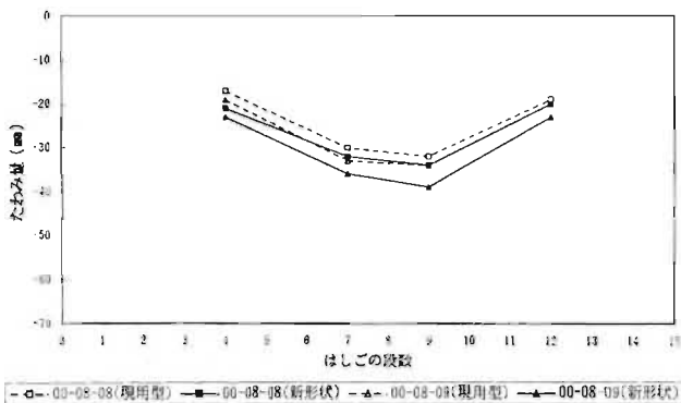
図 2 水平状態のたわみ量の測定結果
