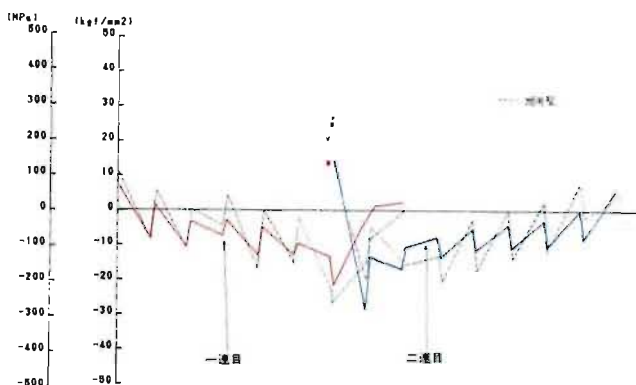
図 3 水平荷重状態の応力測定結果 (784 N (80kgf) 荷重時)
