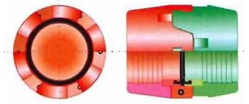
図5 差し込み方式結合金具 (試作2号器)
