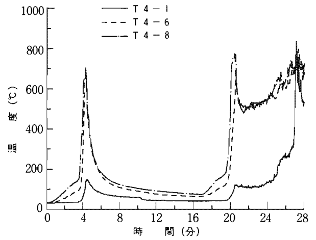
3-2-2 6 畳間 3-2 実験 2
