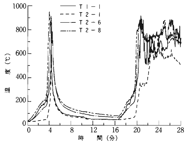
3-2-1 出火室 (4.5 畳間)
