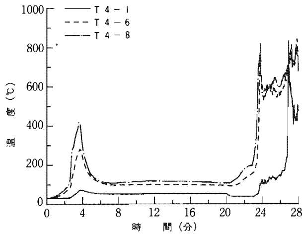
3-1-2 6 畳間 3-1 実験 1
