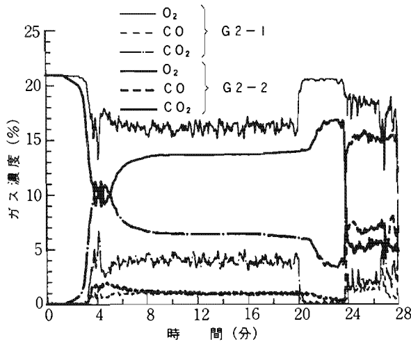
7-1-2 6畳間 7-1 実験1
