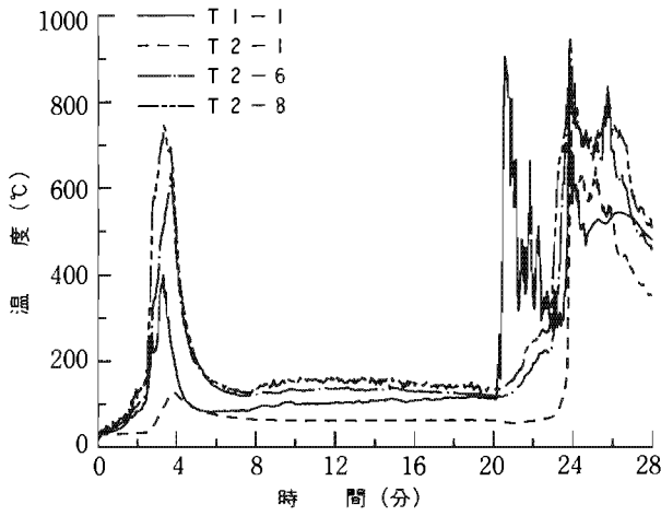
3-1-1 出火室 (4.5 畳間)
