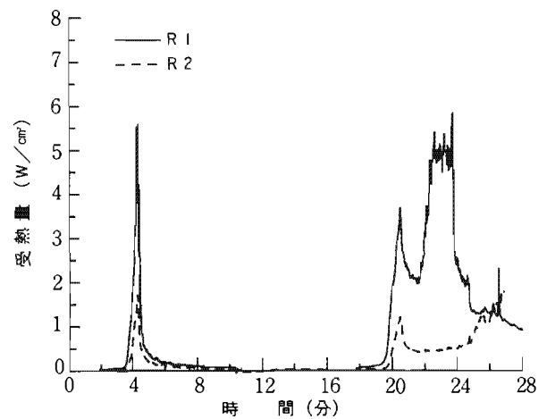
8-2 実験2
