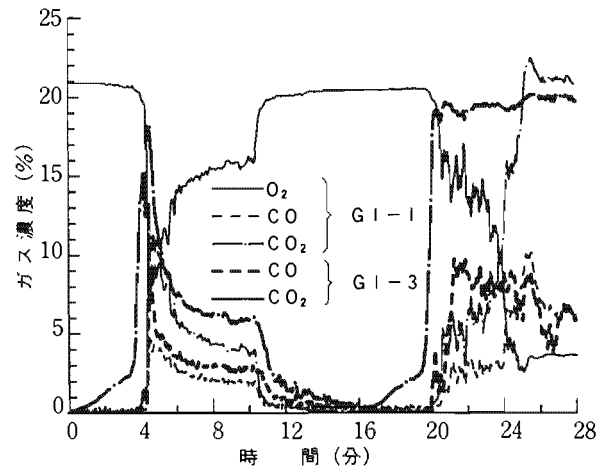
7-2-1 出火室(4.5畳間)
