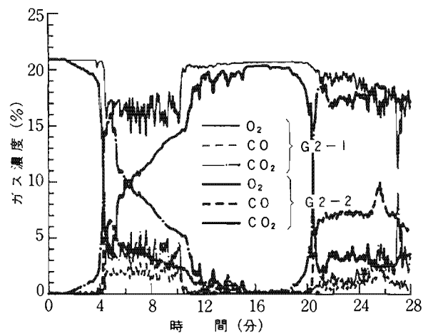
7-2-2 6畳間 7-2 実験2
