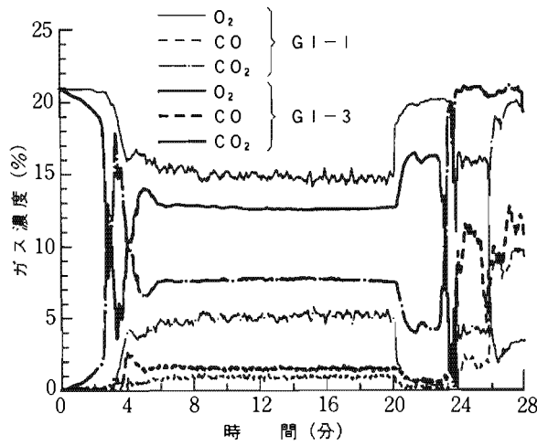
7-1-1 出火室(4.5畳間)
