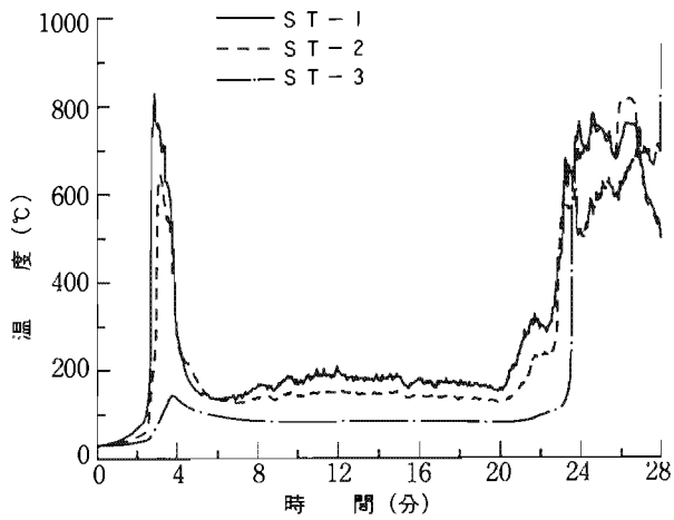
4-1 実験 1
