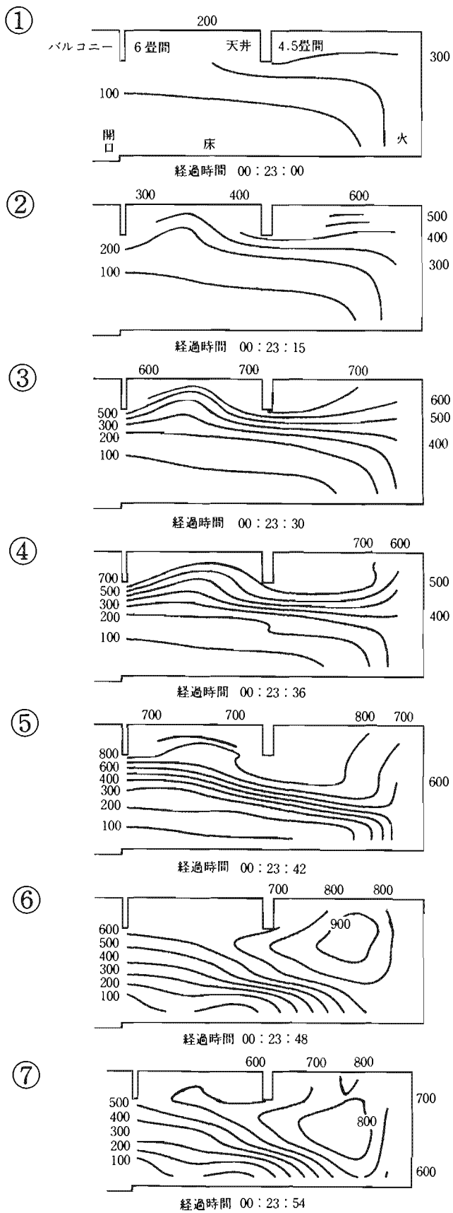
図5 出火室(4.5畳)のフラッシュオーバー発生に伴う火災住戸内温度分布の変化(実験1)
