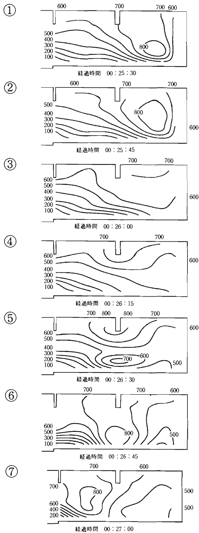
図6 6畳間窓からの火炎噴出に伴う火災住戸内温度分布の変化(実験1)
