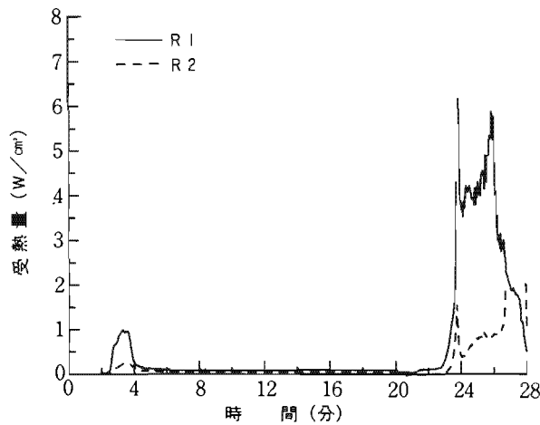
8-1 実験1
