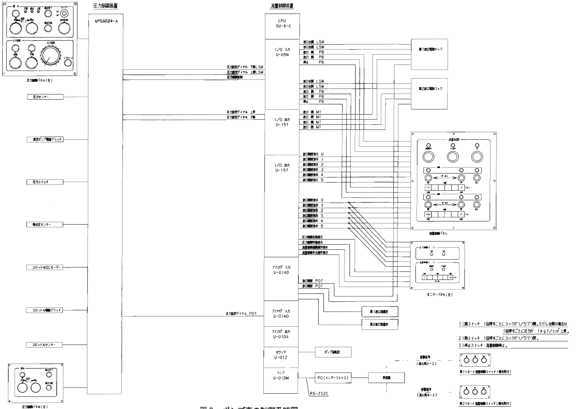
図2 ポンプ車の制御系統図
