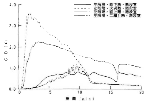
図2 左階段のCO濃度変化 (CASE-1)
