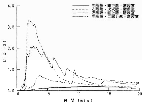
図11 左階段のCO濃度変化 (CASE-4)
