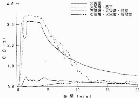
図4 火災階右方向のCO濃度変化 (CASE-4)
