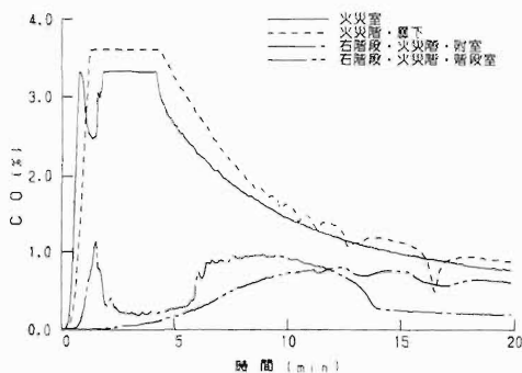
図10 火災階右方向のCO濃度変化 (CASE-3)
