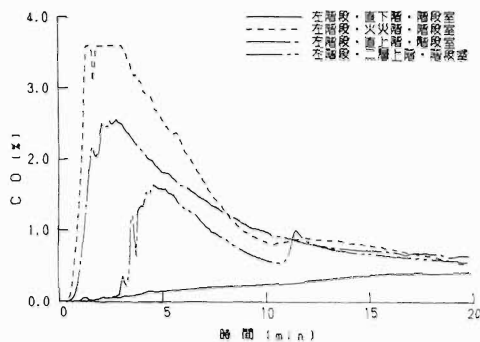
図12 左階段のCO濃度変化 (CASE-3)
