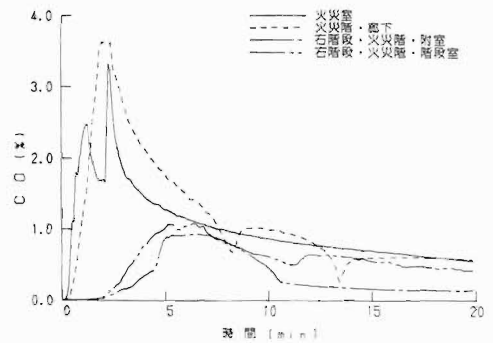
図5 火災階右方向のCO濃度変化 (CASE-6)
