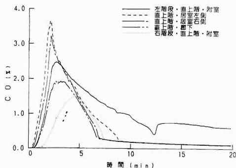
図9 直上階のCO濃度変化 (CASE-5)
