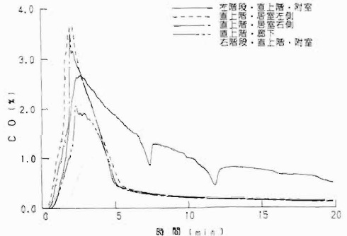
図7 直上階のCO濃度変化 (CASE-6)
