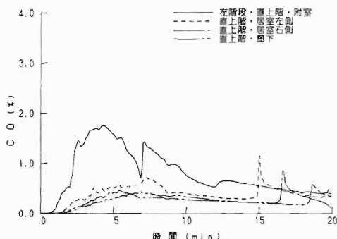
図8 直上階のCO濃度変化 (CASE-4)
