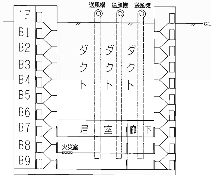
図1-1 実験模型概要図 (立面図)
