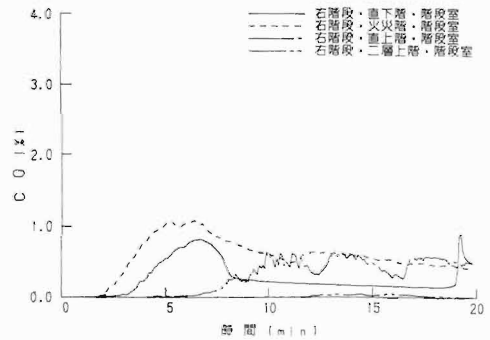
図6 右階段のCO濃度変化 (CASE-6)
