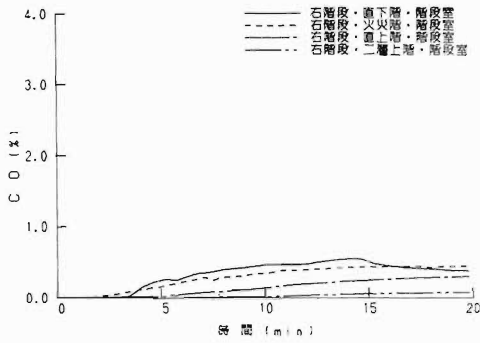
図3 右階段のCO濃度変化 (CASE-1)
