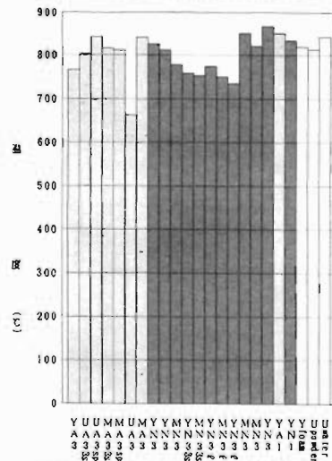
図7 測定点T 2における温度
