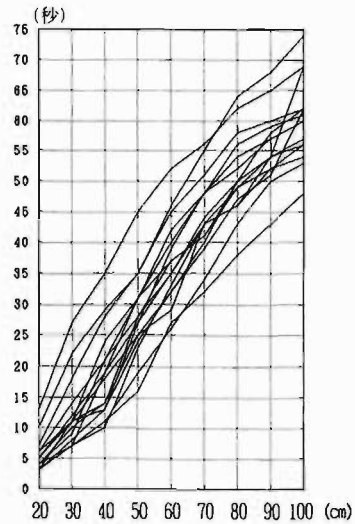
図5 炎の高さと時間の関係
