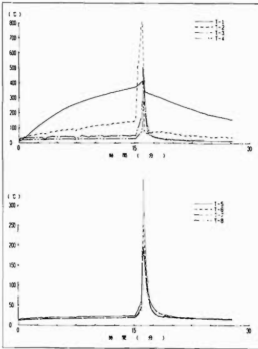
図4 温度測定結果(中性薬剤放射)
