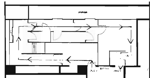
図2 避難経路を明示した平面図
