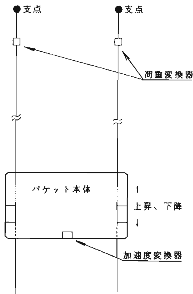
図4 吊りワイヤーロープの張力及びバケットの振動測定方法
