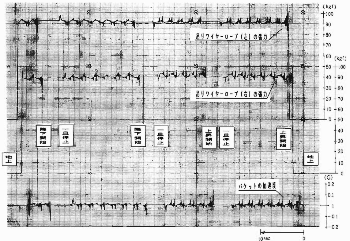
図6 吊りワイヤーロープの張力及び昇降バケットの振動測定結果(積載荷量100kg)
