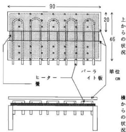
図3 燃焼装置
