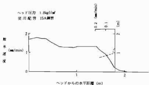
図10 D型ヘッドの散水速度
