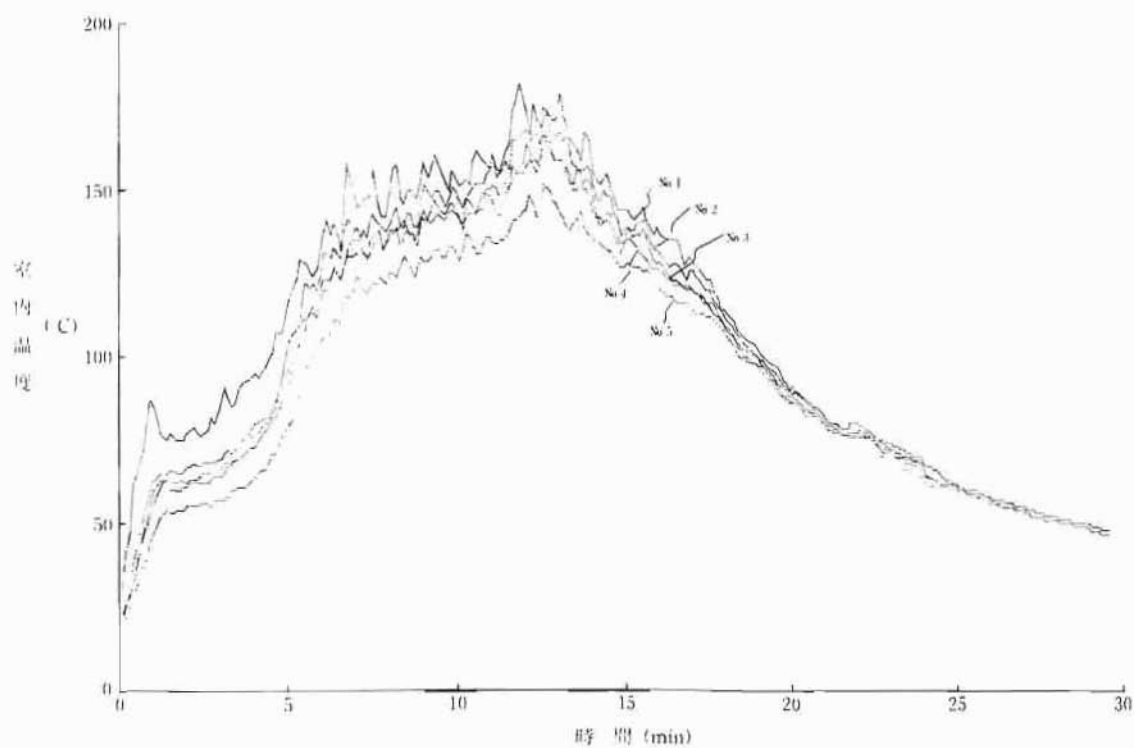
図12 第2消火実験の場合の温度分布
