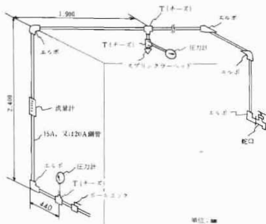
図2 配管概要図
