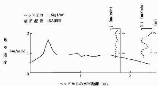
図9 C型ヘッドの散水速度
