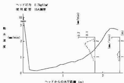
図8 B型ヘッドの散水速度
