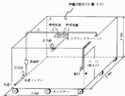
図1 住宅用スプリンクラー模擬実験室
