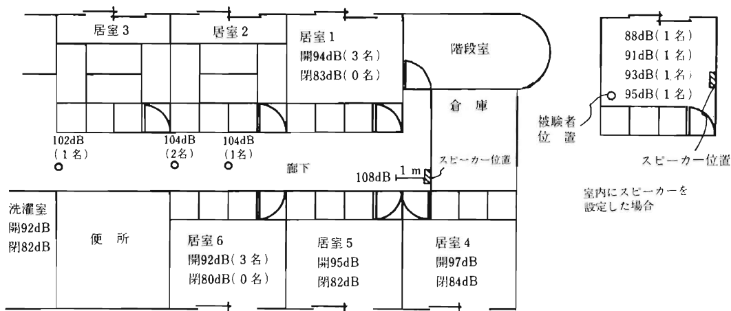
廊下にスピーカーを設定した場合
