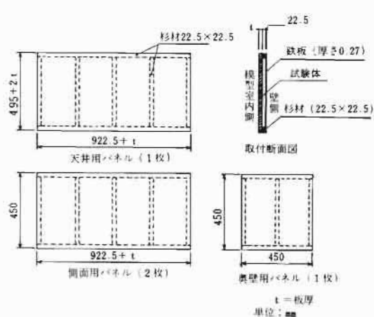
図3 試験体の取付方法
