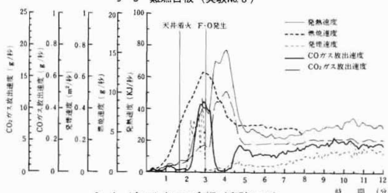
図9 燃焼による諸特性値の変化 (その1)
