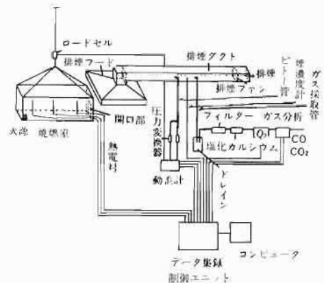
図1 実験装置概要図
