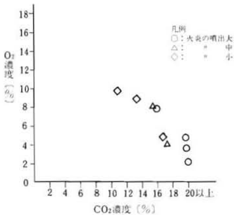
図10 火炎噴出程度別「O 2 -CO 2 」相関図
