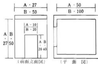
図1 模型燃焼室の概要図
