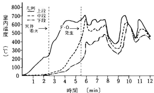
図4 実験No. 8の温度変化
