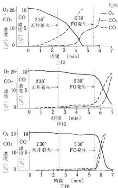
図5 実験No.8のガス濃度変化
